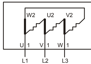
Połączenie w trójkąt
